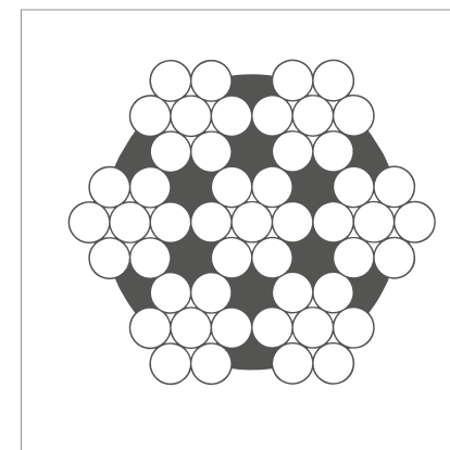
Aufbau Litze kabel / Drahtseil 7x7
